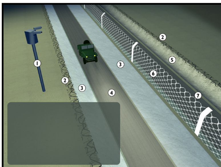
Diagrama del Cerco de Seguridad en Cisjordania: 1.- Cámaras de vigilancia, 2.- Alambre de espino, 3.- Arena fina, 4.- carretera pavimentada, 5.- cuneta 1,8 a 2,4 m, 6.- valla 3 m, 7.- camino de tierra.
